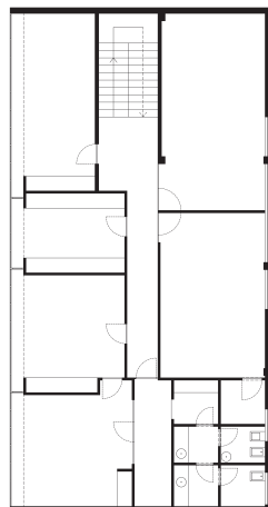
1º Andar
